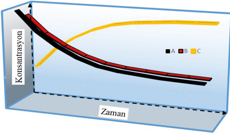
Şekil 3.1. Reaktiflerin ve ürünlerin konsantrasyonlarının zamanla değişimi
